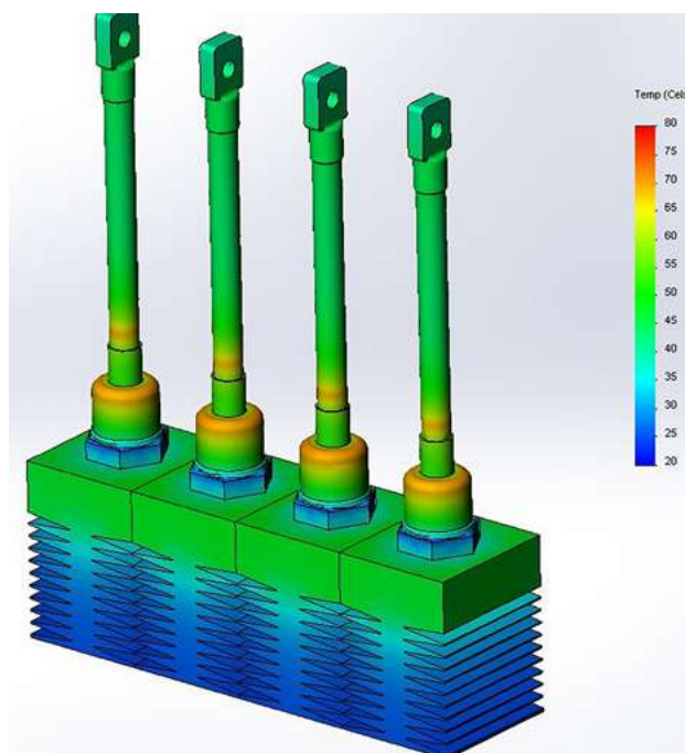
Рис. 4. Нагрев при исправном режиме работы
