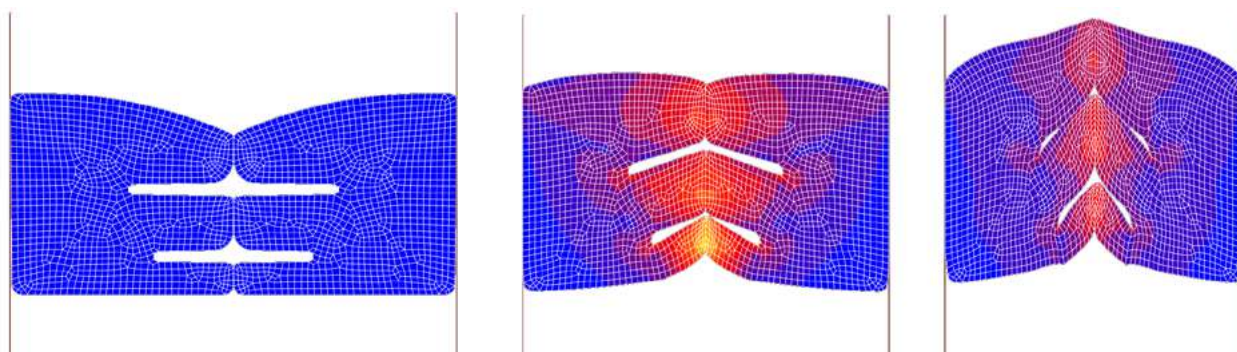
Рис. 8. Деформация элемента с тремя парами устойчивости
