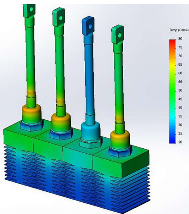
Рис. 6. Нагрев при обрыве одного диода
