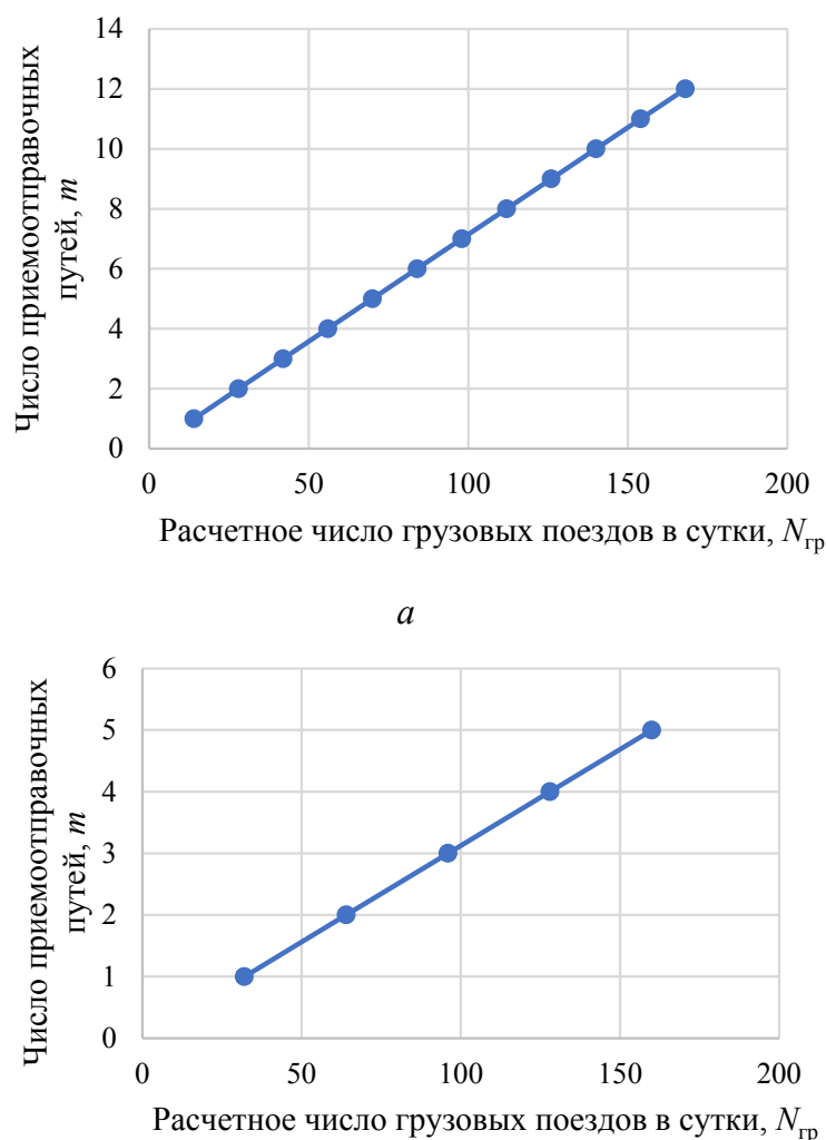
Рис. 2. Зависимость числа приемоотправочных путей от расчетного числа грузовых поездов при продолжительности технологического «окна» 75 мин: а — смена локомотива; б — смена локомотивной бригады
