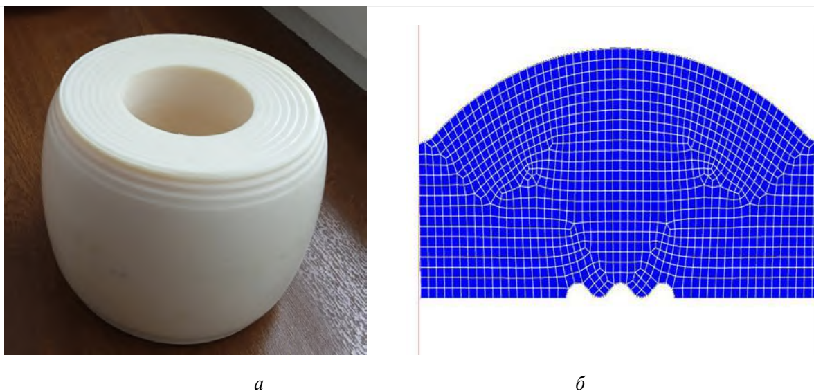
Рис. 3. Опорный полимерный элемент поглощающего аппарата ПМКП-110:
