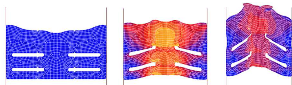
Рис. 6. Деформация трехсоставного полимерного элемента
