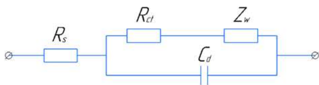
Рис. 1. Схема Рендлса как пример схемы ячейки
