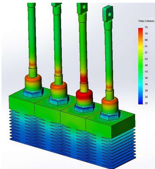
Рис. 5. Нагрев при пробое одного диода
