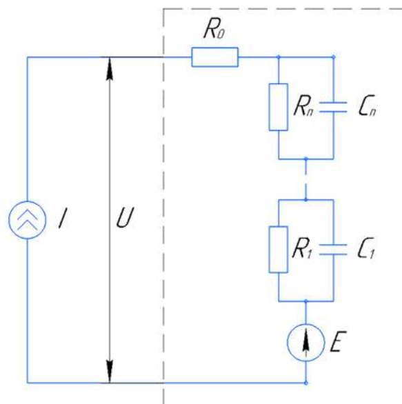
Рис. 4. \Gamma -образная схема замещения ЛИА
