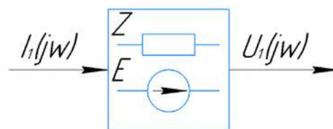
Рис. 3. Двухполюсник ЛИА, представленный как «черный ящик»
