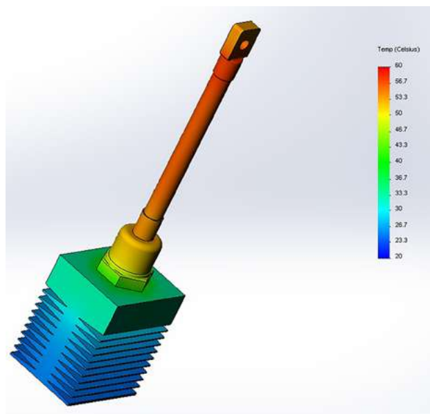
Рис. 3. Модель нагрева одного диода
