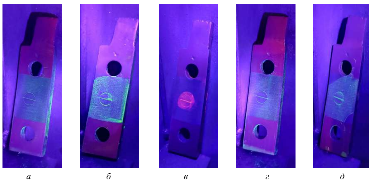
Рис. 5. Дефектограмма стопорной планки при УФ-освещении (светлая поверхность): a — MR76F; б — КСФ12; в — Mi-GLOW850; г — Magnaglo 14HF; д — Диагма-1613
