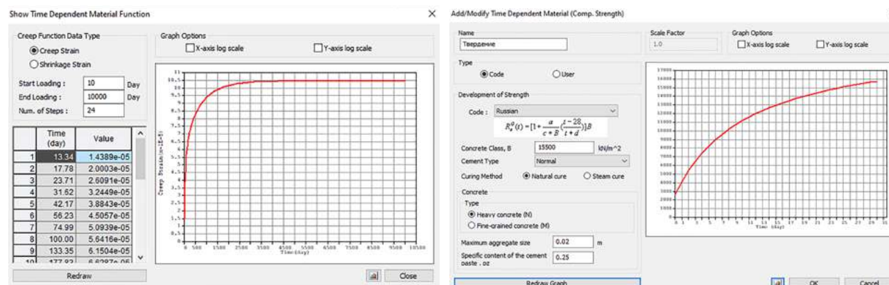
Рис. 10. Графики изменений свойств бетона по времени
