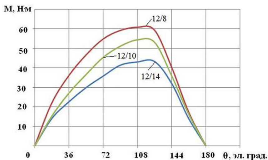
Рис. 2. Характеристики электромагнитного момента M_{\text{э}} = f(\theta) для магнитных систем ВВД различной конфигурации в насыщенном режиме работы
