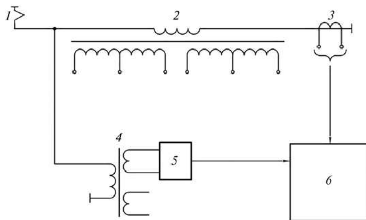
Рис. 2. Схема измерений:
