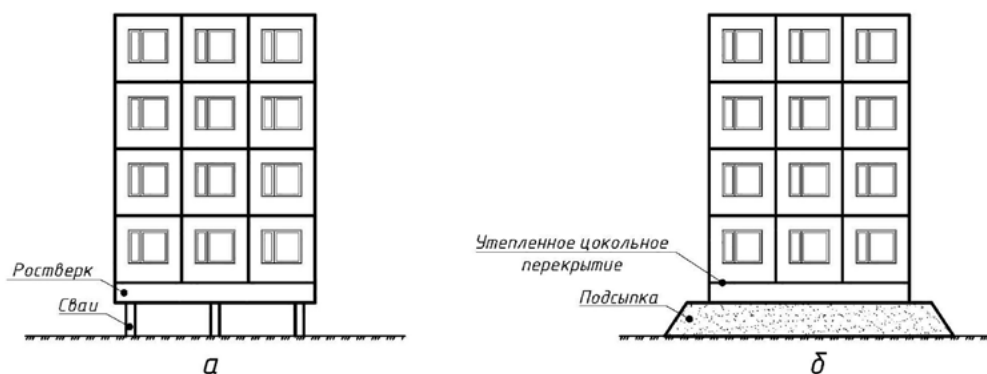
Рис. 1. Способ сохранения грунтов основания в мерзлом состоянии с использованием высокого свайного ростверка с проветриваемым подпольем (а) и подсыпки (б)
