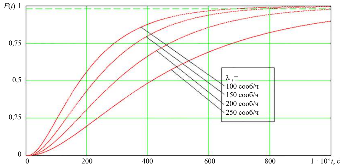
Рис. 2. Вид функции распределения времени передачи сообщений в радиосети с общим каналом связи
