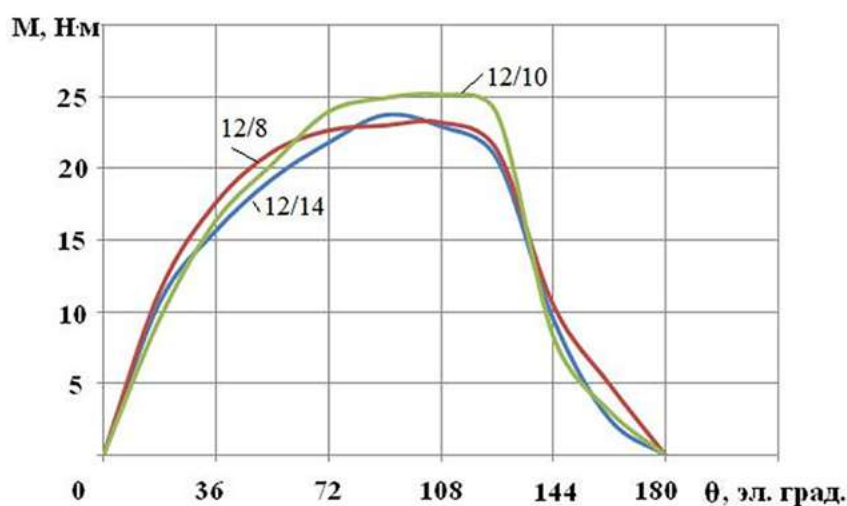
Рис. 3. Характеристики электромагнитного момента M_{\text{э}} = f(\theta) для магнитных систем ВВД различной конфигурации в ненасыщенном режиме работы
