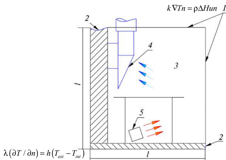
Рис. 2. Область решения:
