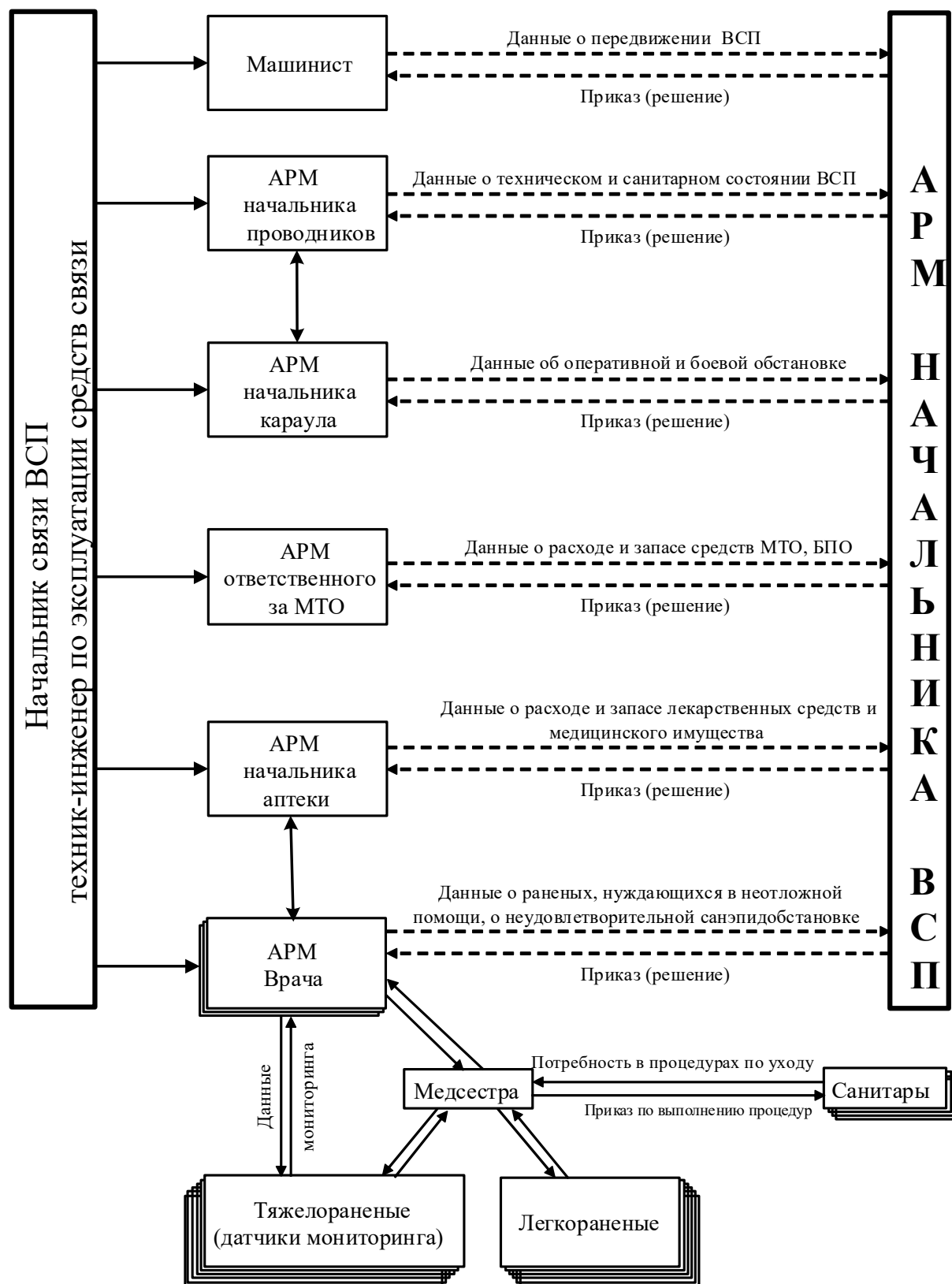
Рис. 2. Перспективная модель обмена «внутренней» информацией в ВСП
