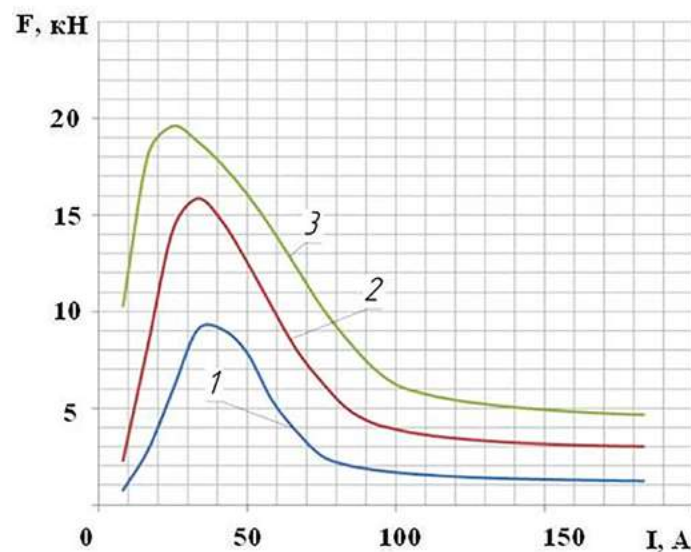
Рис. 7. Результаты расчета сил ОМП при совпадении зубцов и вертикальном смещении ротора по оси Y на: 1 — 0,3 мм; 2 — 0,6 мм; 3 — 0,9 мм
