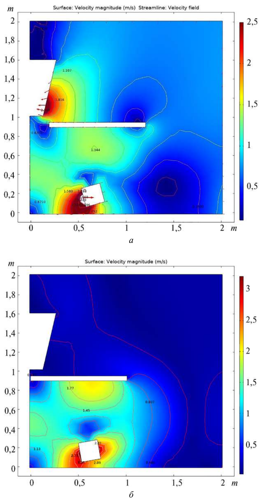
Рис 4. Поля скоростей:
