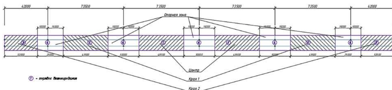
Рис. 8. Стадийность бетонирования
