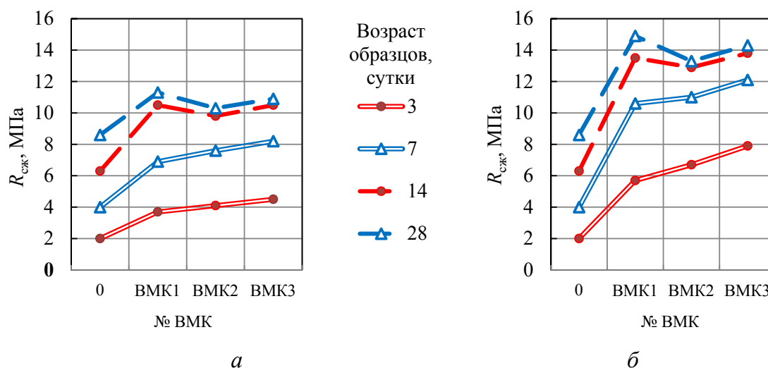
Кинетика изменения прочности на сжатие камня из гипсоизвесткового вяжущего, модифицированного ВМК разного химического состава: при количестве ВМК в смеси вяжущего: а — 10 мас.%; б — 20 мас.%
