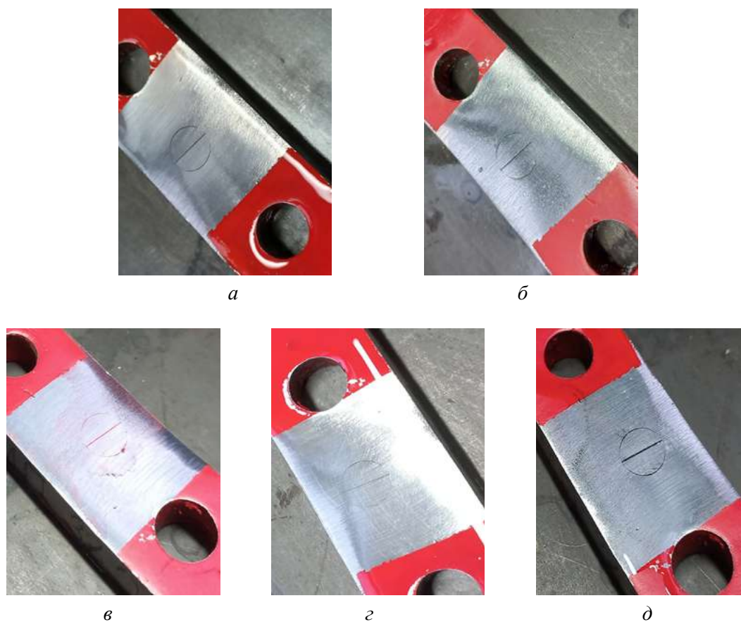
Рис. 4. Дефектограмма стопорной планки при дневном освещении (светлая поверхность): a — MR76F; б — КСФ12; в — Mi-GLOW850; г — Magnaglo 14HF; д — Диагма-1613
