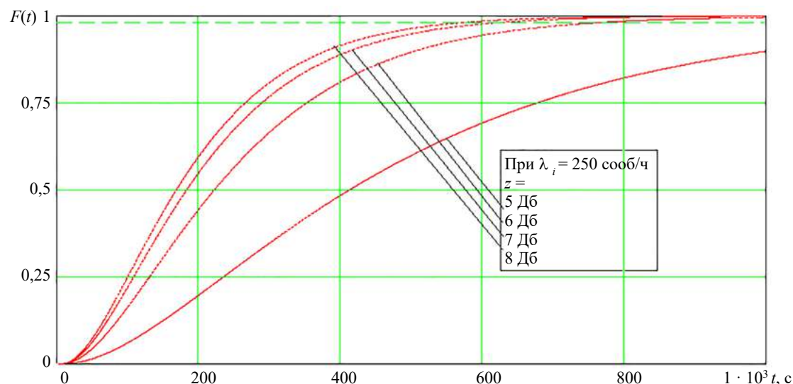
Рис. 3. Вид функции распределения времени передачи сообщений в зависимости от отношения сигнал/шум в радиосети с общим каналом связи
