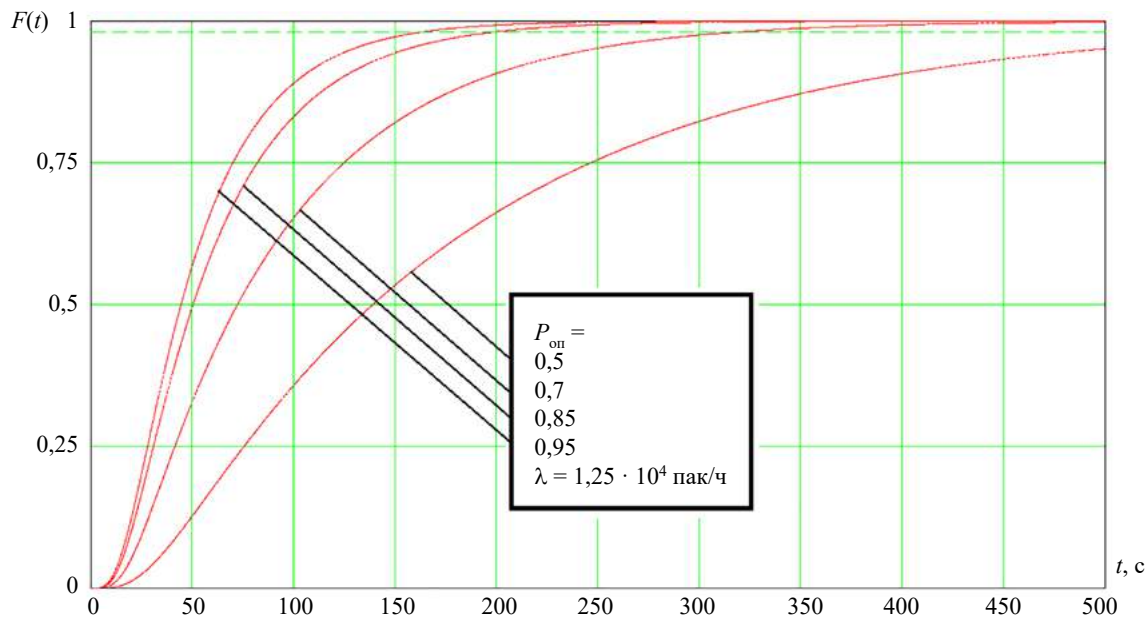
Рис. 4. Вид функции распределения времени передачи пакета данных в зависимости от вероятности успешного приема
