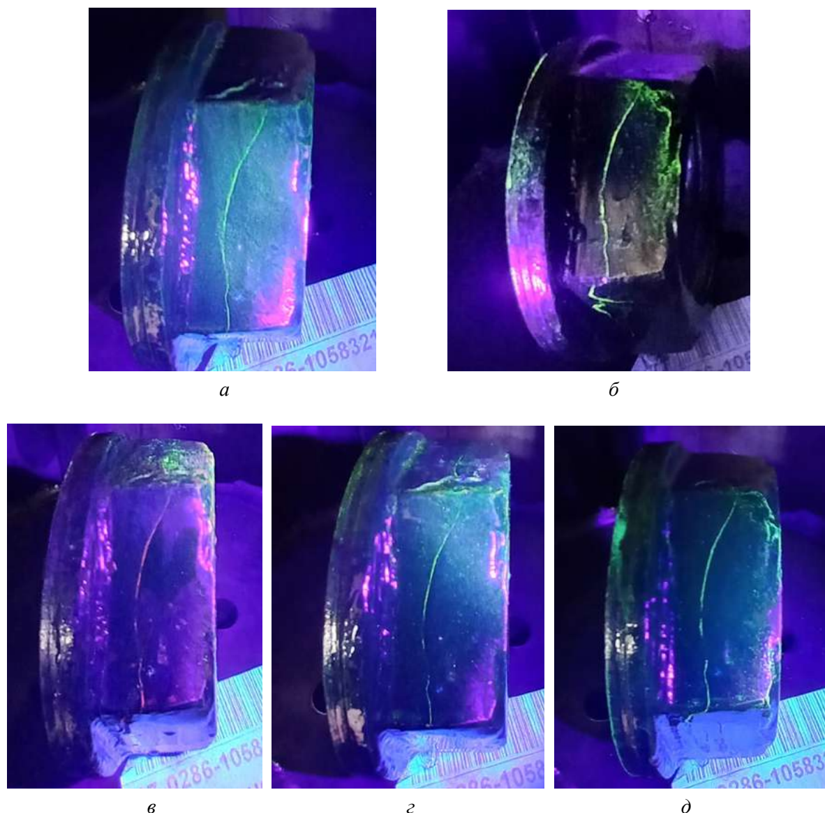
Рис. 2. Дефектограмма гайки шестигранной с фланцем поводка тележки (темная поверхность с нанесением лакокрасочного покрытия толщиной до 20 мкм в виде черной краски из распылительного баллона): а — MR76F; б — КСФ12; в — Mi-GLOW850; г — Magnaglo 14HF; д — Диагма-1613
