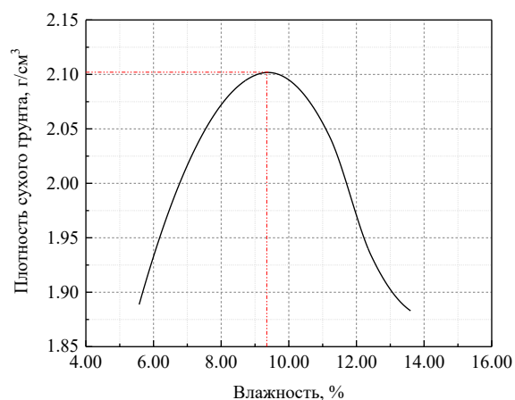
Рис. 3. Зависимость плотности грунта от влажности
