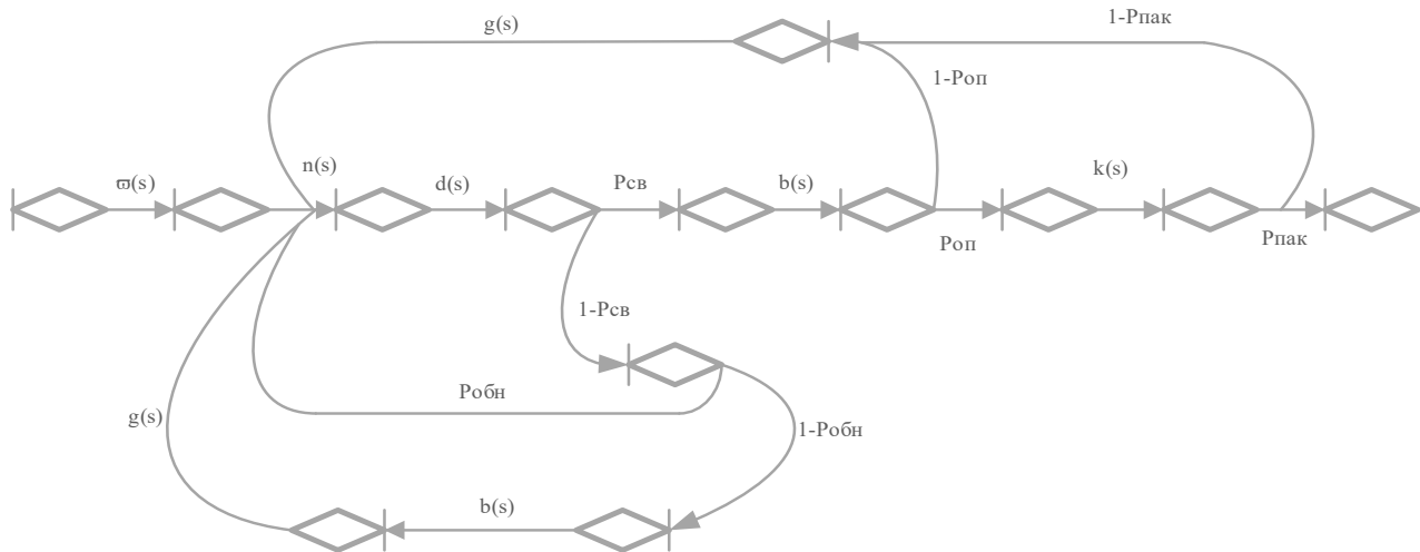
Рис. 1. Стохастическая сеть функционирования сети ПРС с общим каналом связи:
